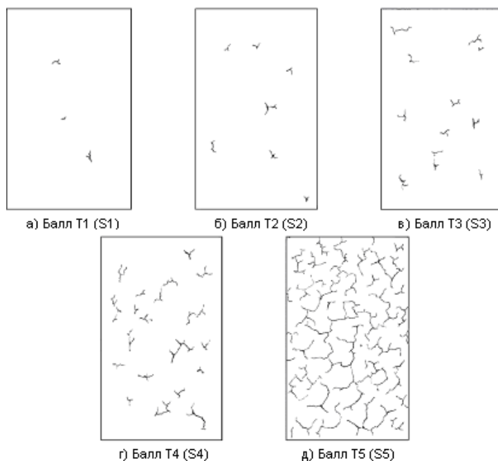
Рисунок А.1 – Растрескивание без предпочтительного направления (площадь осматриваемой поверхности от 1 до 2 дм 2 )
